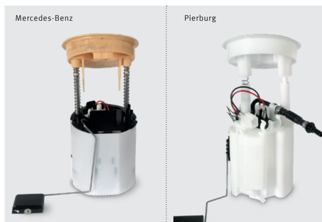
Fig. 1 : comparaison des modules d'alimentation en carburant
