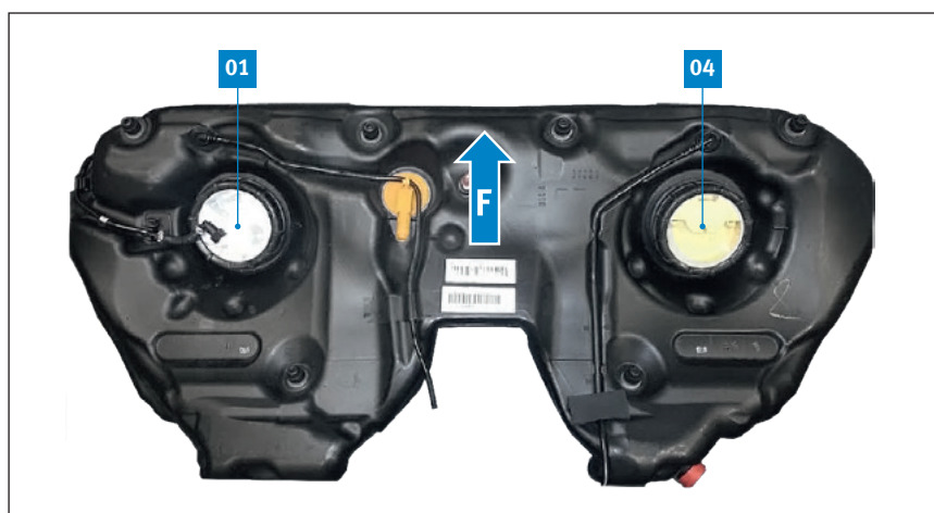
Fig. 4 : réservoir de carburant (vue de dessus)
