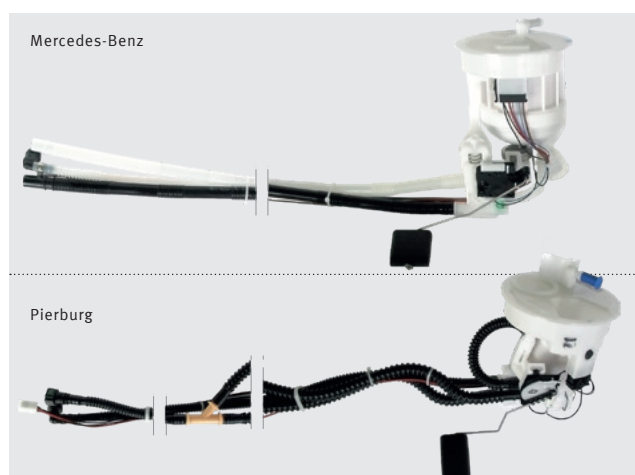
Fig. 2 : comparaison des unités d'indicateur de niveau
