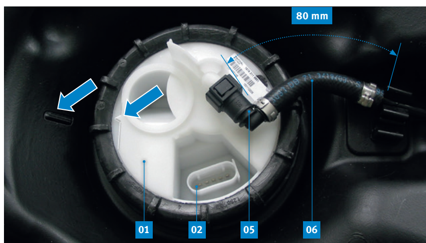
Fig. 5 : couvercle à bride de l'unité d'indicateur de niveau
